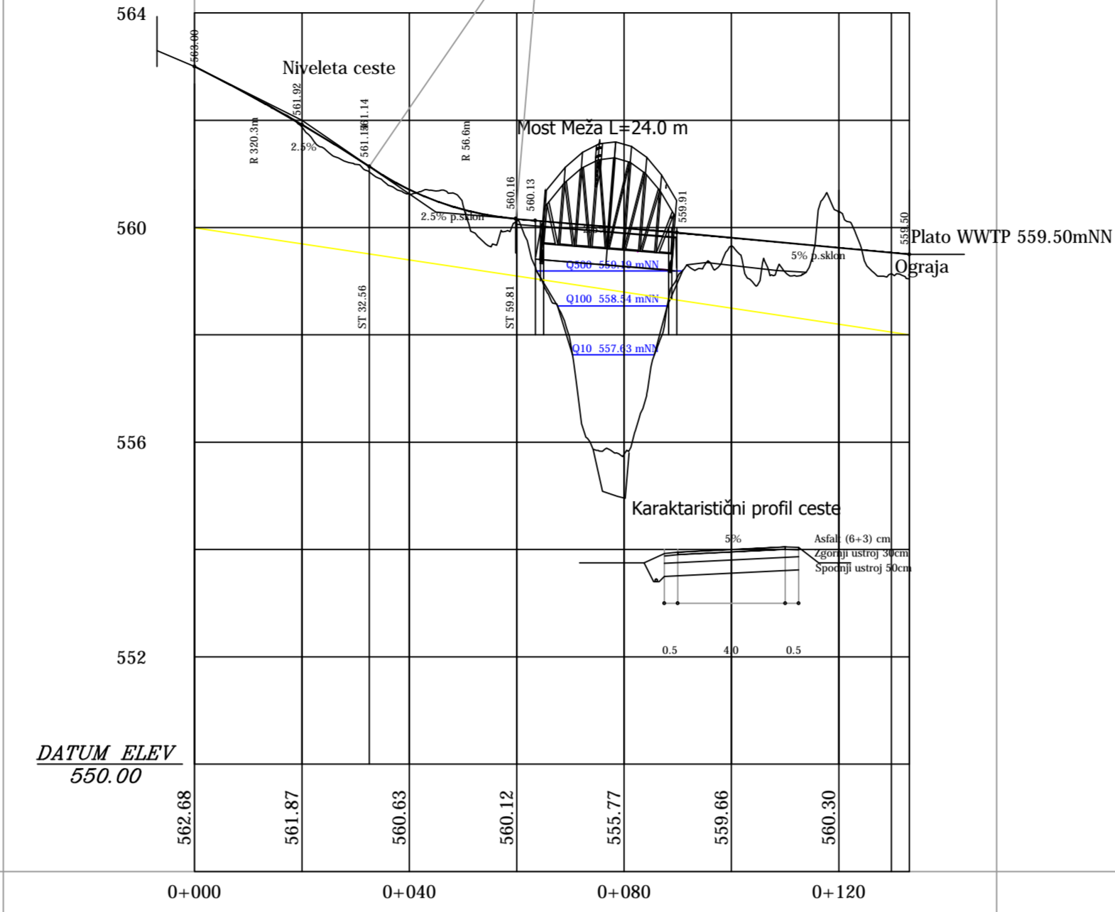
Dovozna cesta L=129.8m in most na ČN Črna
