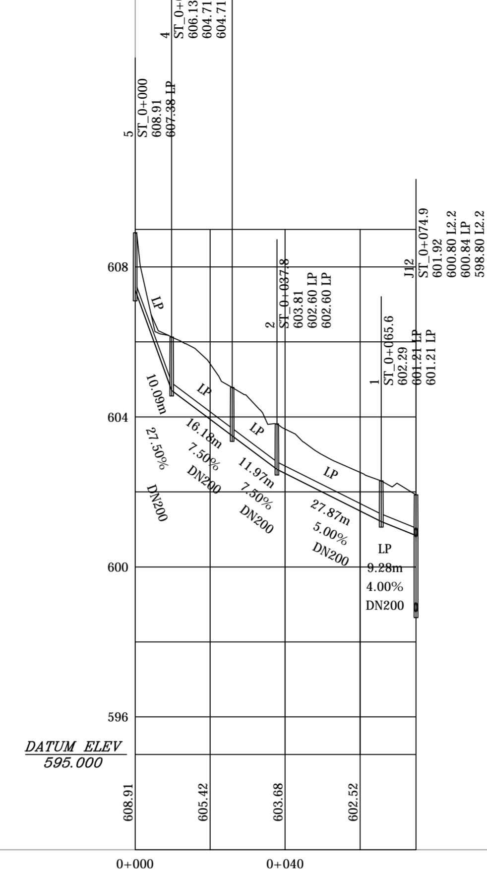
Kanal LP Črna DN200 74.9m
